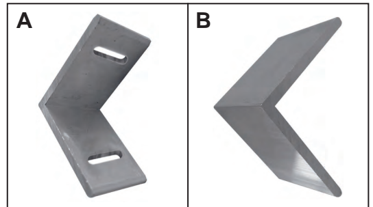
A. 2214 ΓΩΝΙΑ ΣΥΝΔΕΣΕΩΣ ΧΑΜΗΛΩΝ ΟΔΗΓΩΝ JOINT CORNER FOR LOW DRIVERS B. 2014 ΓΩΝΙΑ ΣΥΝΔΕΣΕΩΣ ΧΑΜΗΛΩΝ ΟΔΗΓΩΝ JOINT CORNER FOR LOW DRIVERS
